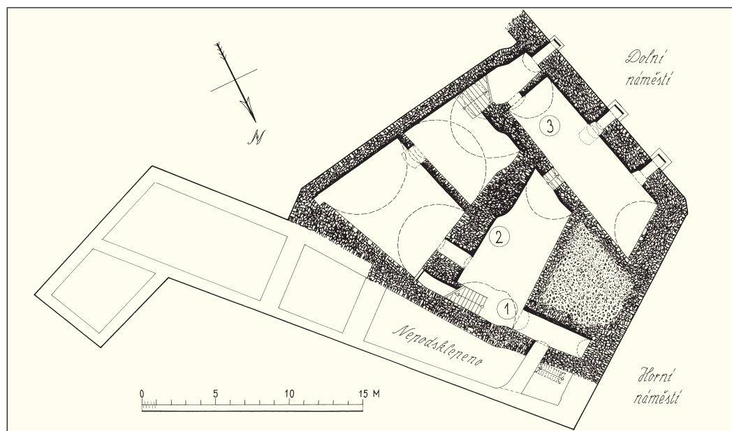
Plánek sklepení Horní náměstí 16, dům U zlatého jelena. (Podle stavebně-historického průzkumu překreslil P. Zlinský, 2009.)
